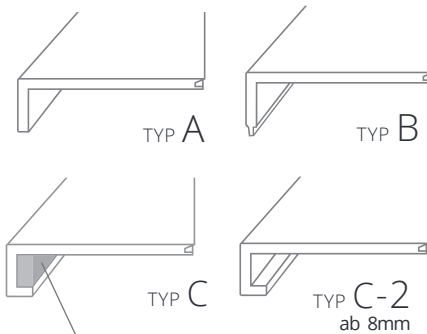
Wersseitige VERSTÄRKUNG bei Belägen bis 7,9mm
